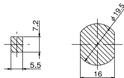
カム穴あけ寸法
